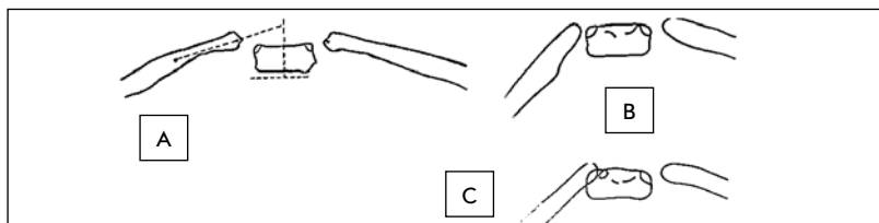
Рис. 22. Признаки Mehta
